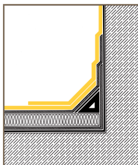
Cant Strip op isolatie met tweelaagse dichting.
