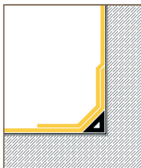
Cant Strip op niet-geïsoleerde dakvloer
